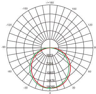
LS-5EHB240W-50K
