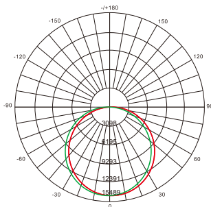
LS-5EHB200WHV-50K
